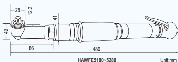
HAWFE5180~5280
